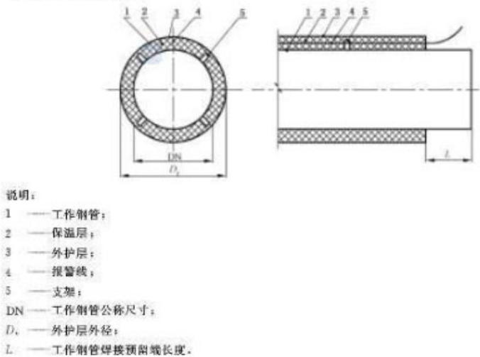
图 1 产品结构示意图
