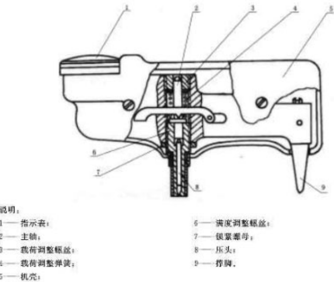
图 B.1 巴氏硬度计结构示意图
