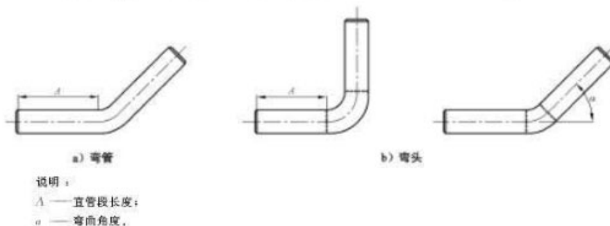
图 2 弯头与弯管示意图
